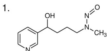
4-(Methylnitrosamino)-1-(3-pyridyl)-1-butanol (NNAL)
